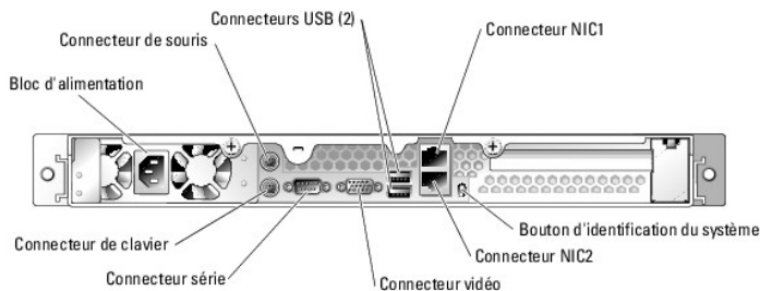
Figure 1-2. Caractéristiques et voyants du panneau arrière
